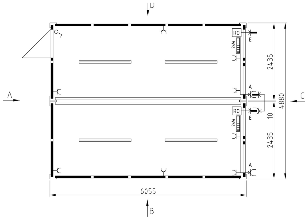
Ansicht B
