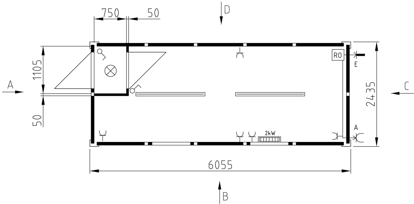
Ansicht A
